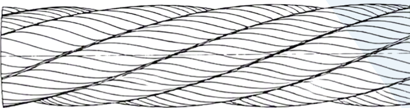
Rope Lay Right Hand Regular Lay (Z Lay)
